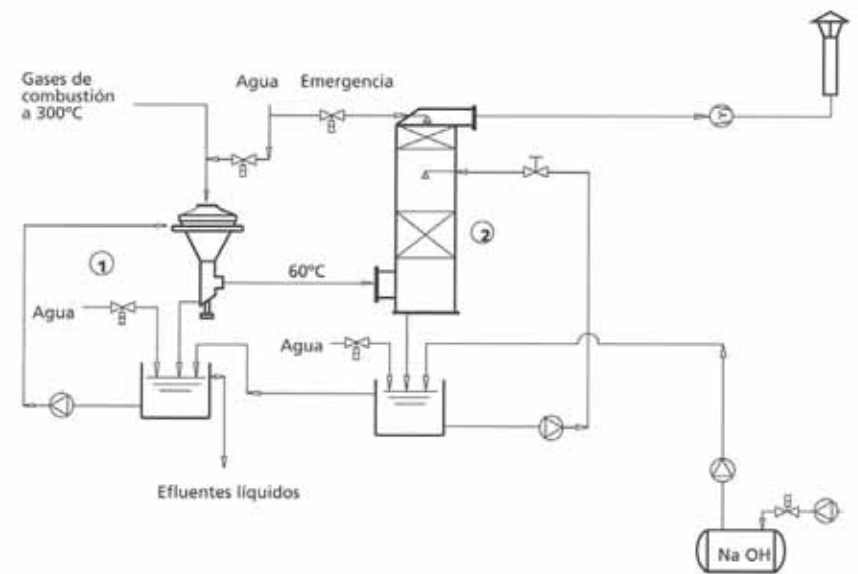
Fig. 17-5. Esquema de tratamiento de los gases. Módulo 1: Quench. Módulo 2: Scrubber con dosaje de Na OH.
