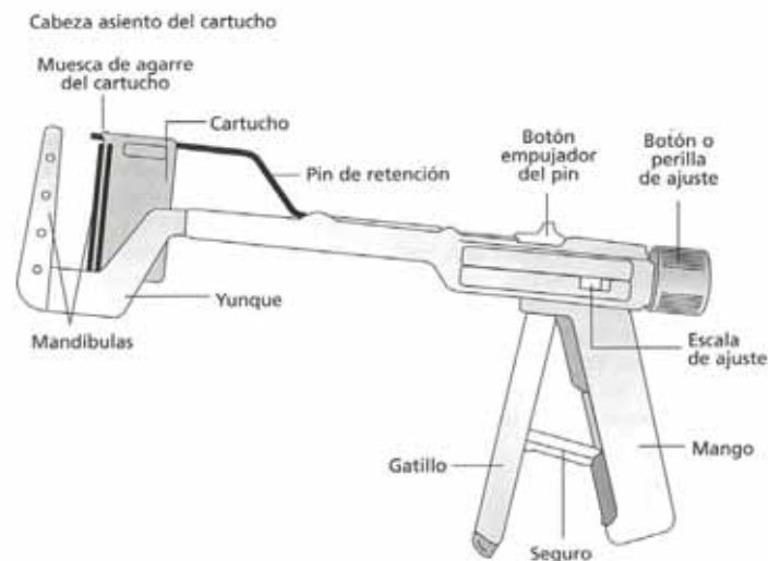
Fig. 8-20. Descripción de una engrapadora lineal.
