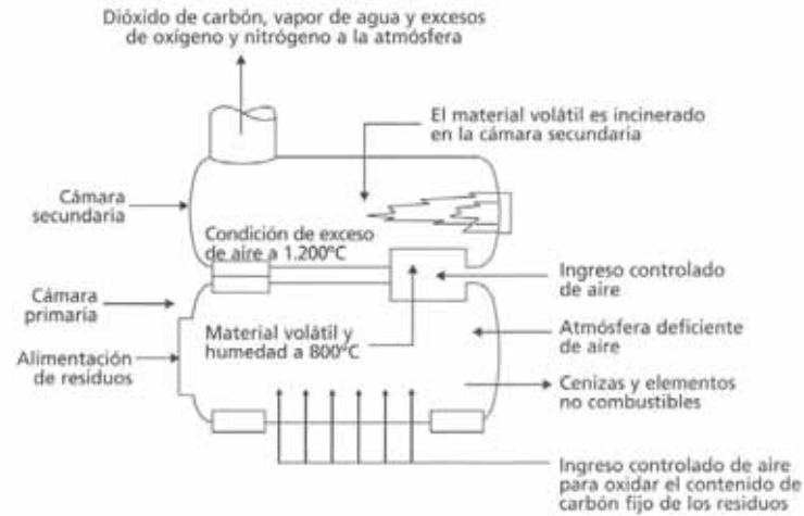
Fig. 17-4. Horno pirólítico. Descripción de las cámaras primaria y secundaria.
